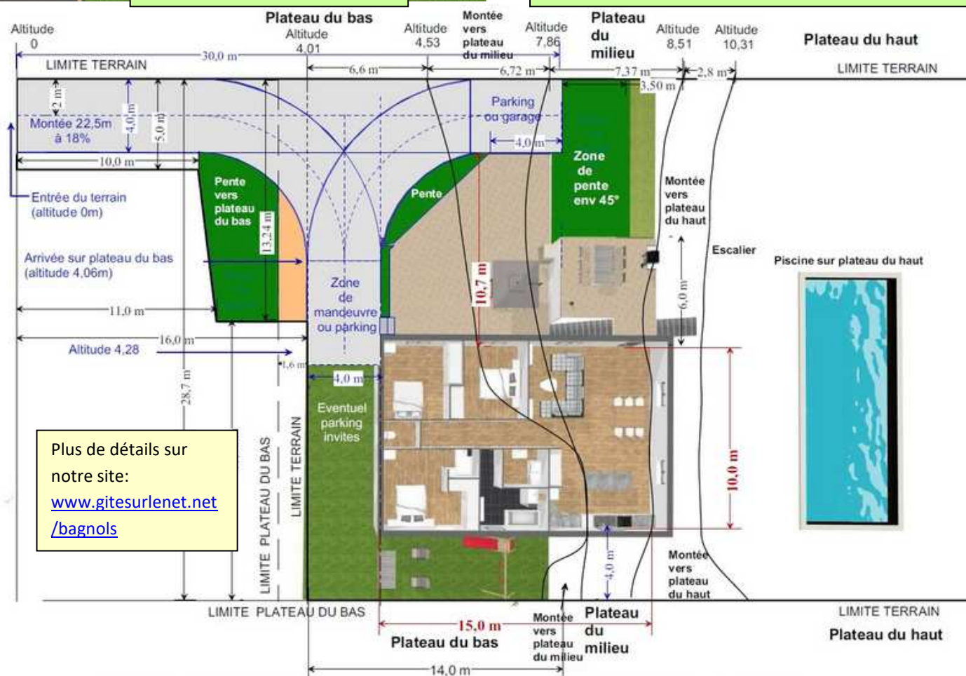
PLAN 14-1: ETUDE IMPLANTATION MAISON DOUBLE SUR LE PLATEAU DU BAS (vue de dessus)
