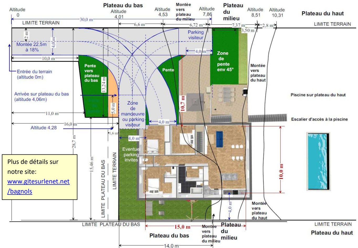
PLAN 14-2: ETUDE IMPLANTATION MAISON AVEC GARAGE SUR LE PLATEAU DU BAS (vue de dessus)
